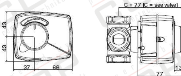
2 pont, 24 V (ARA6x8 előreszerelt segédkapcsolóval)
